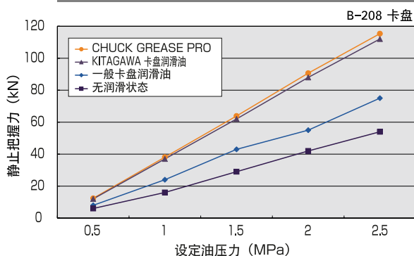
图1 使用润滑脂的情况下夹持力比较
