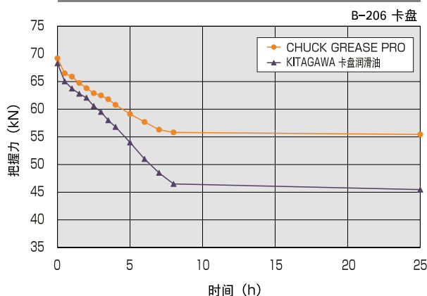
图2 不同卡盘润滑脂所引起的的夹持力低下比较
